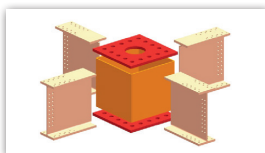
DRUM-RCS構法の接合部金物
